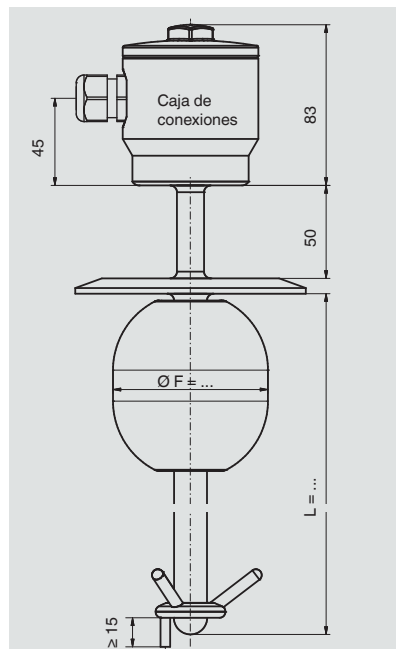
Con conexión de tubo soldada
