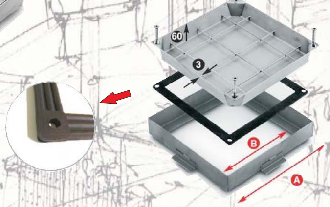
Tapa de registro rectangular
